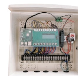
制御ノード
